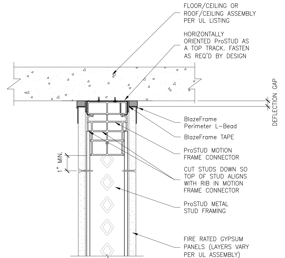
SECTION A-A
