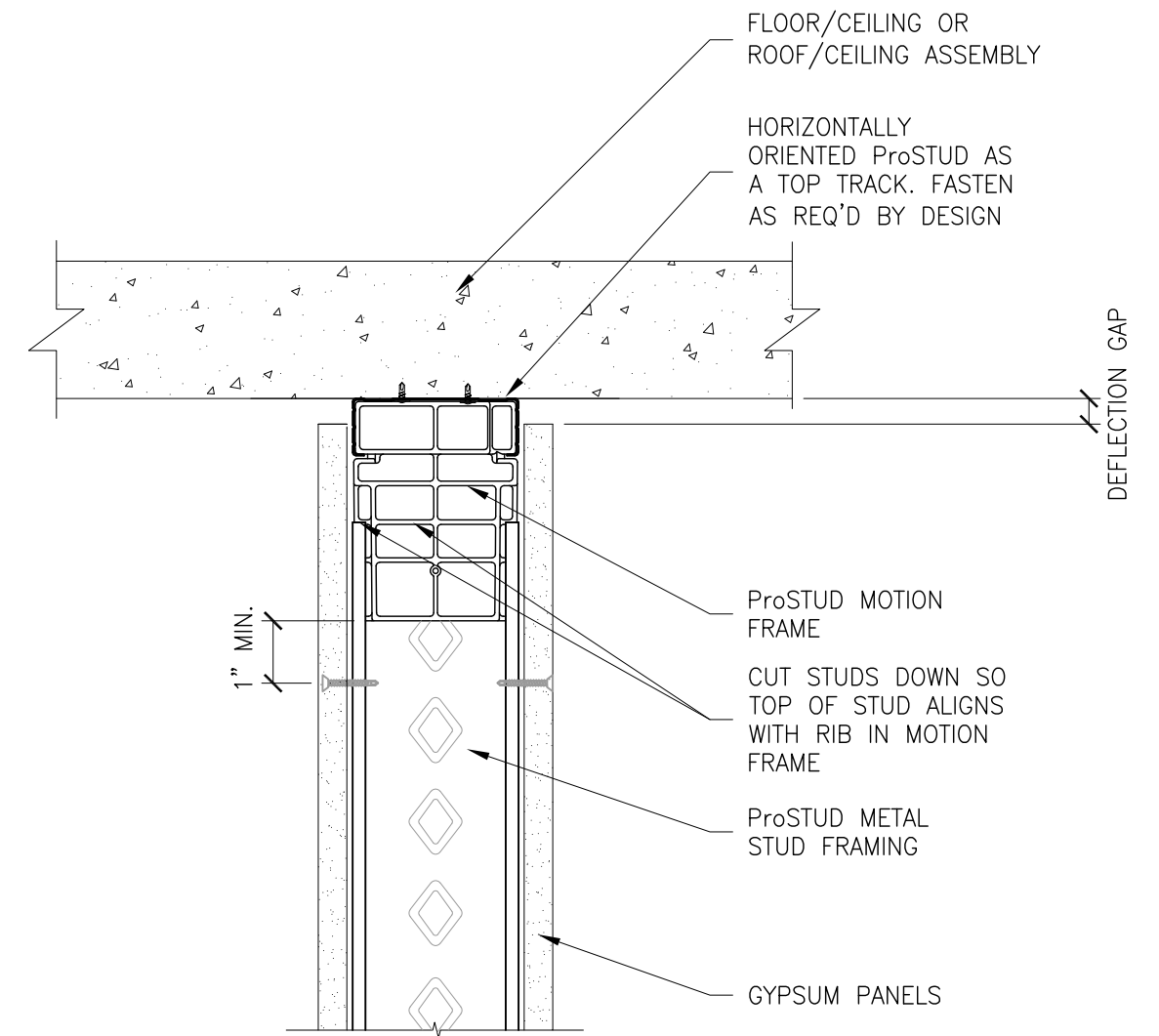
SECTION A-A
