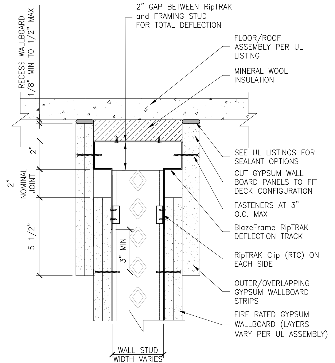
SECTION A-A
