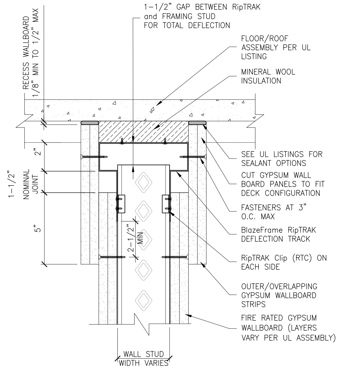
SECTION A-A
