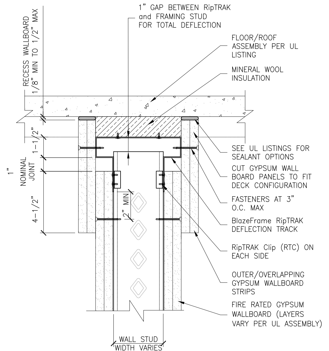
SECTION A-A
