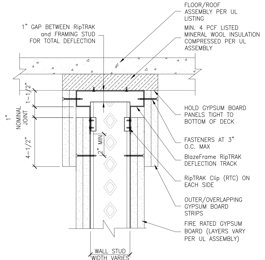
SECTION A-A
