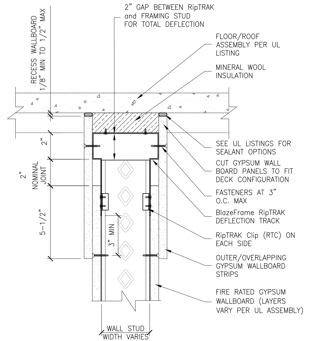
SECTION A-A
