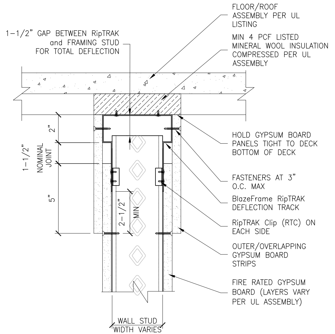
SECTION A-A
