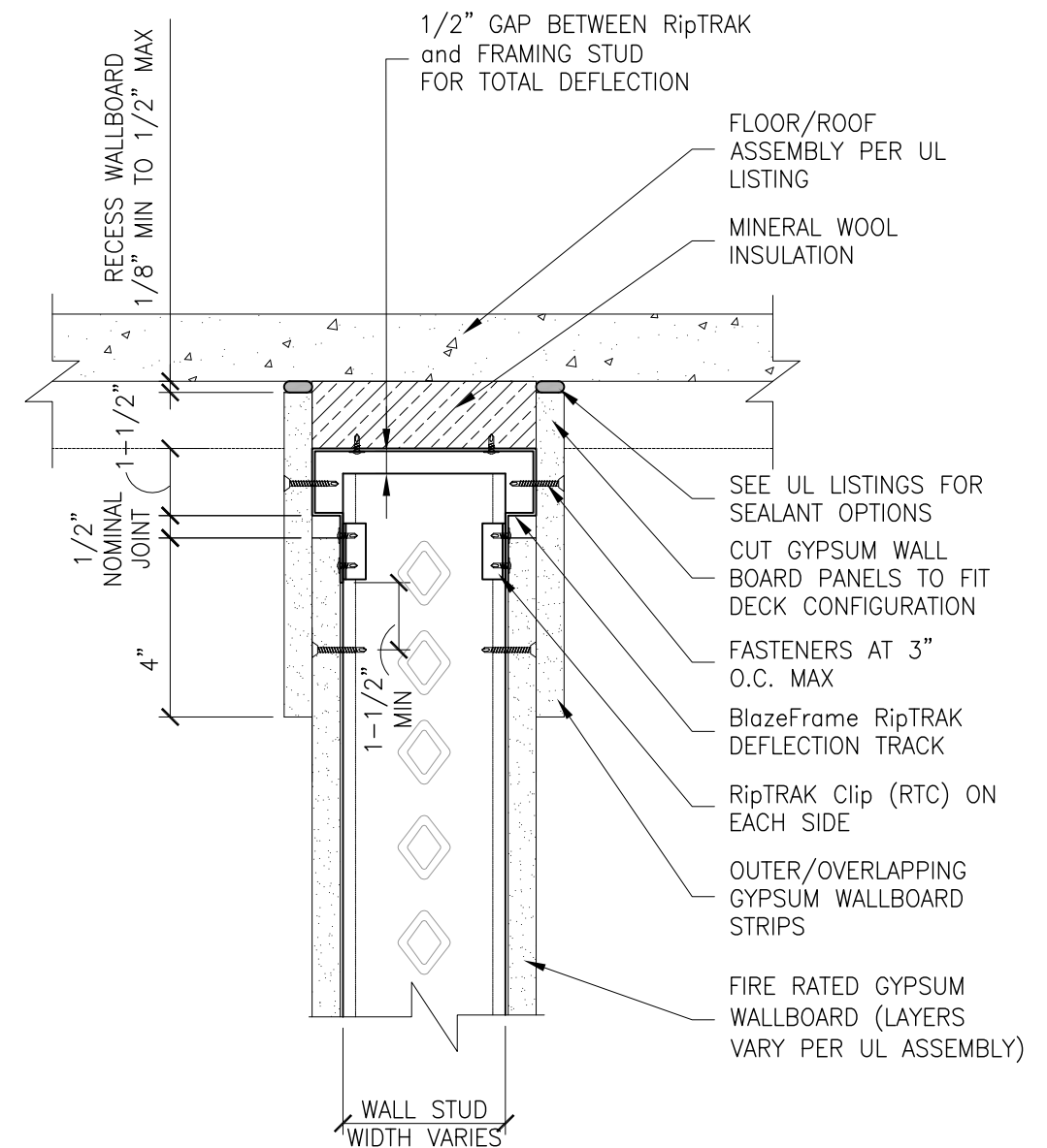
SECTION A-A
